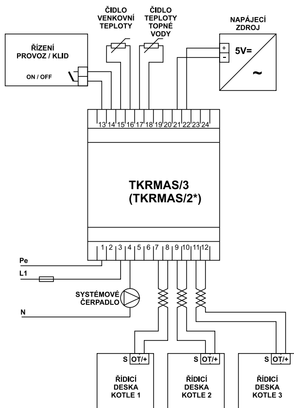
Schéma zapojení pro ekvitemní regulaci kaskády
